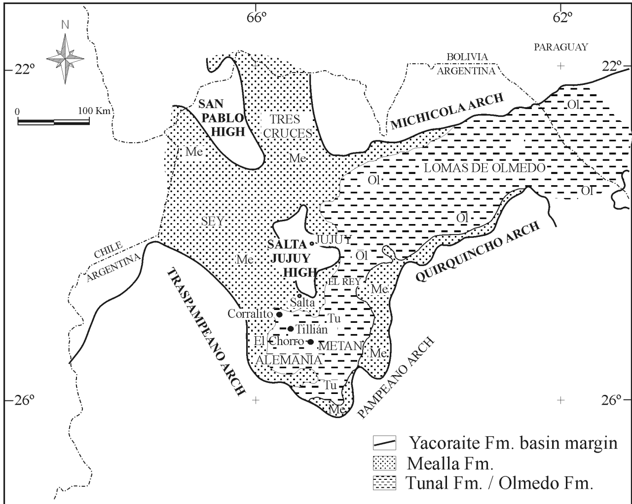
Figure 3. Stratigraphic units overlying the Yacoraite Formation (adapted from Salfity and Marquillas, 1994) / unidades estratigráficas sobrepuestas a la Formación Yacoraite (adaptado de Salfity y Marquillas, 1994).
